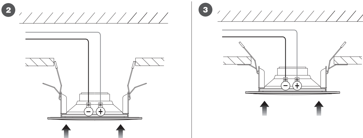
Zusammenbau der Lautsprecher
